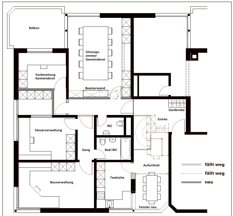
Grundriss 1. Obergeschoss neu
